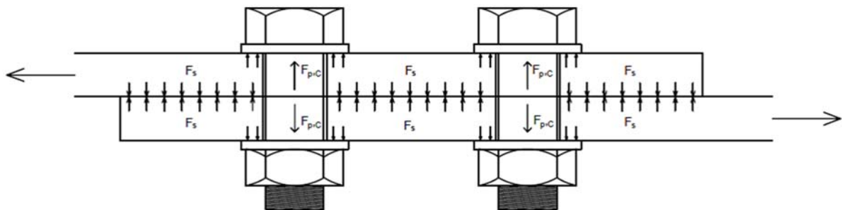
Slika 3.17 Spoj limova s visokovrijednim vijcima
