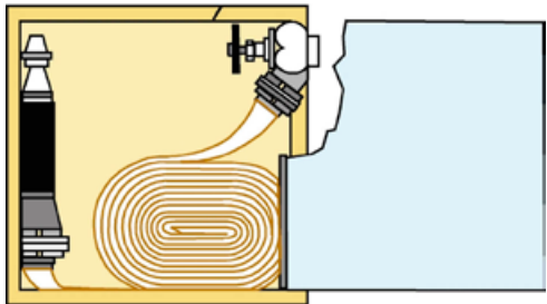
Sl. 58. Zidni unutarnji hidrantski ormarčić sa ventilom, crijevom i mlaznicom. Dužina jednog vatrogasnog crijeva iznosi 15 metara.
